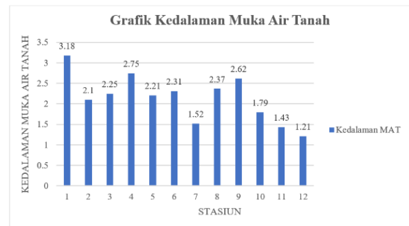
Gambar 6. Grafik Kedalaman Muka Air Tanah
