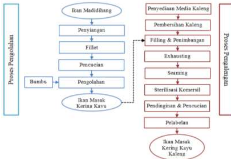
Gambar 1. Proses pengolahan dan pengalengan ikan tuna kering kayu
