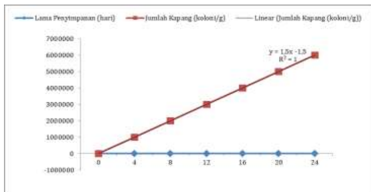
Gambar 4. Grafik pendugaan jumlah mikroba reaksi orde nol
